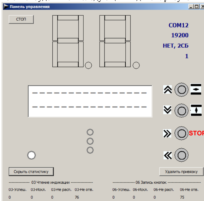
Рисунок И.16 – Вид окна УПУ при отсутствии ответов от целевого ВИМУ (статистика выведена)
