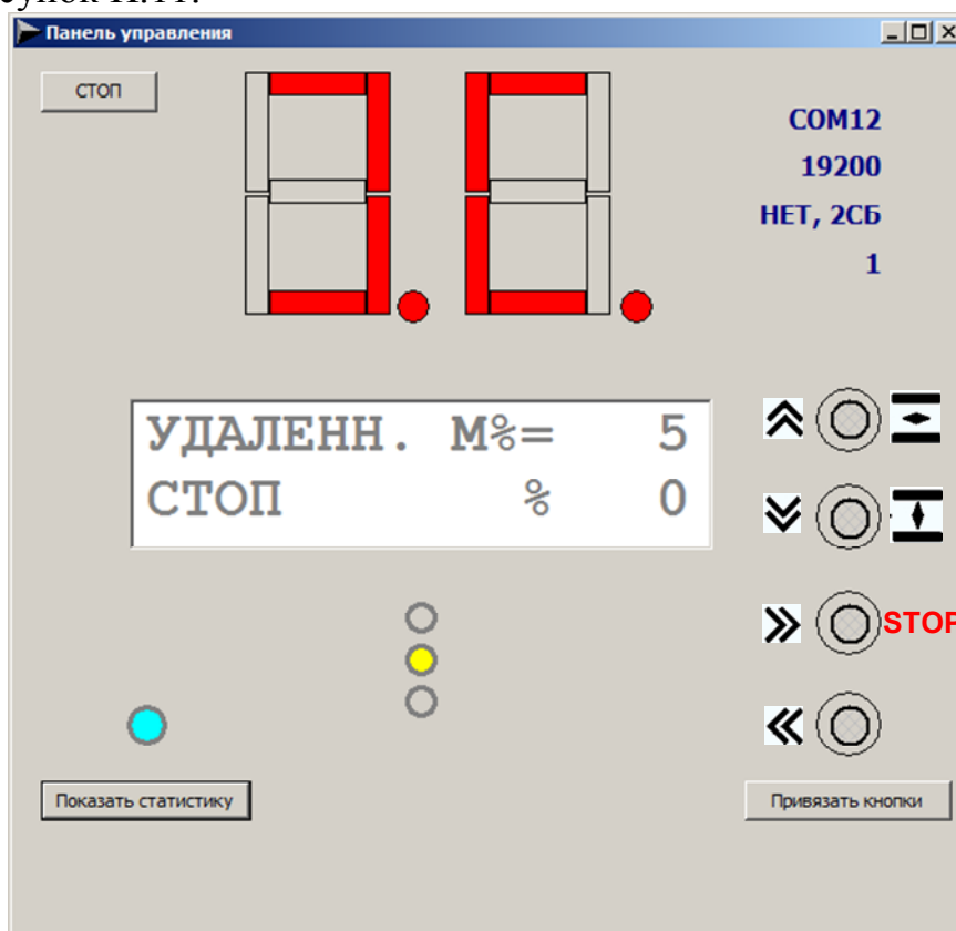
Рисунок И.11 – Окно УПУ после установления связи с ВИМУ
