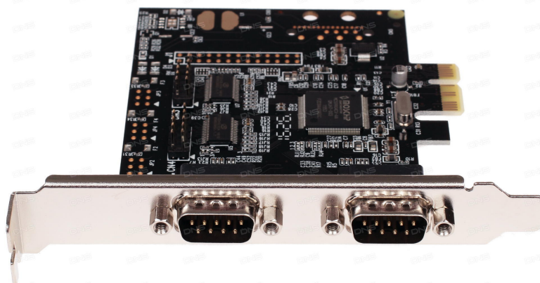
Рисунок И.1 – Контроллер Espada FG-EMT04A-1
