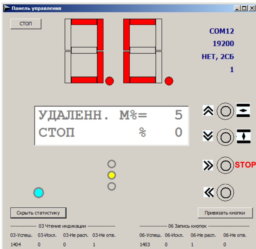
Рисунок И.13 – Окно УПУ с включенным отображением статистики
